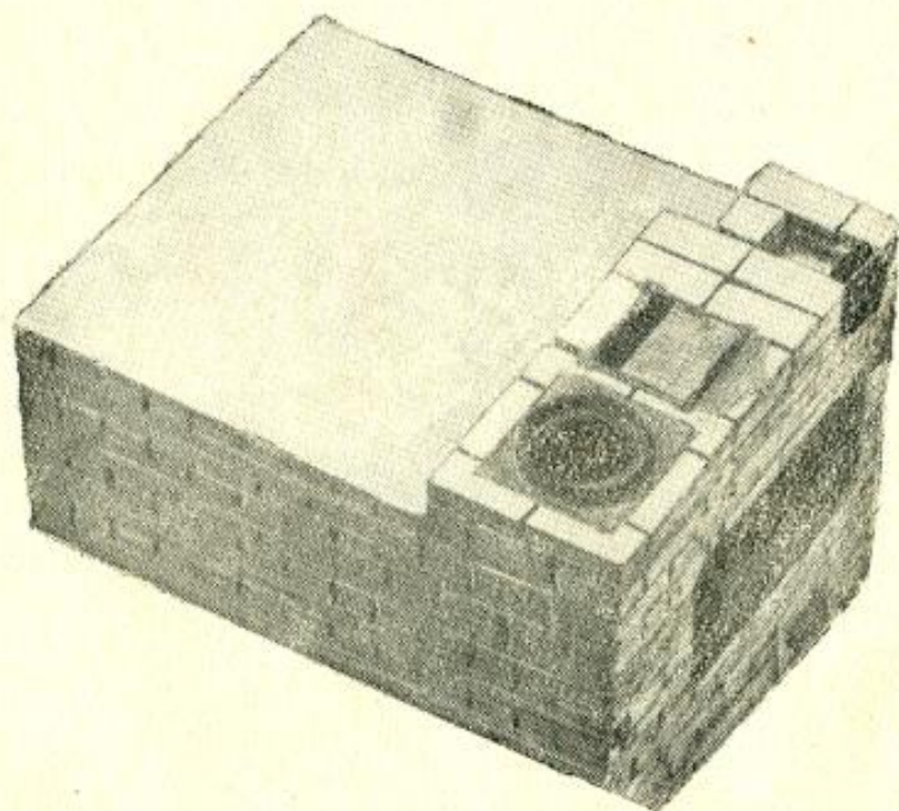
Рис. 38. Кладка 24-го ряда.
