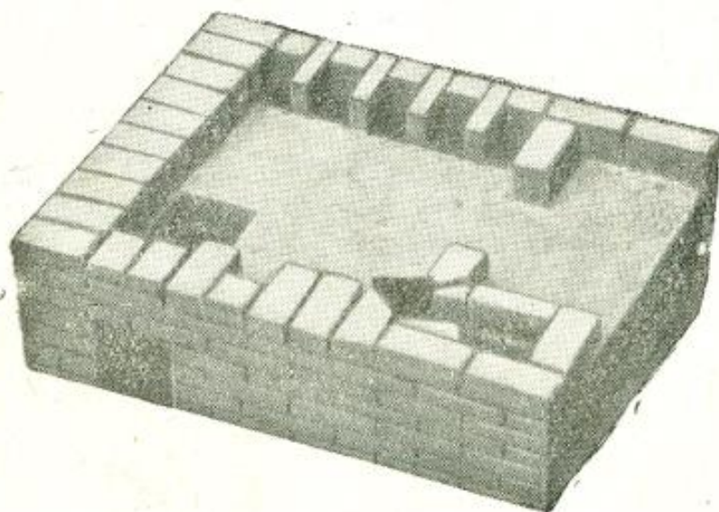
Рис. 27 Кладка 14-го ряда.
