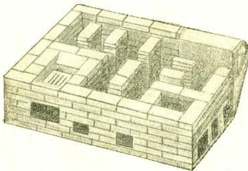
Рис. 21. Кладка 7-го ряда.
