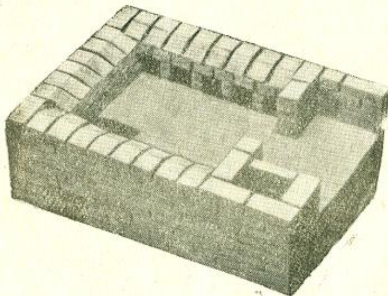
Рис. 30. Кладка 16-го ряда.
