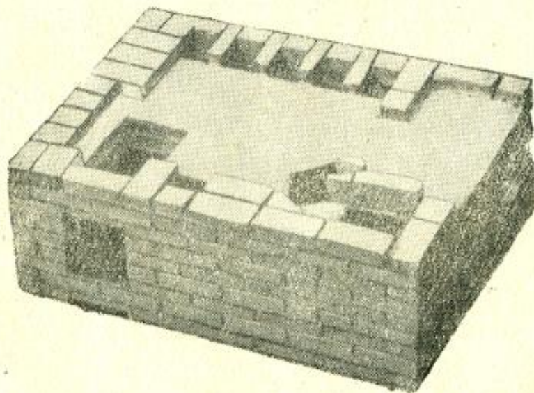
Рис. 27. Кладка 13-го ряда.
