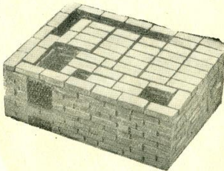
Рис. 26. Кладка 12-го ряда.
