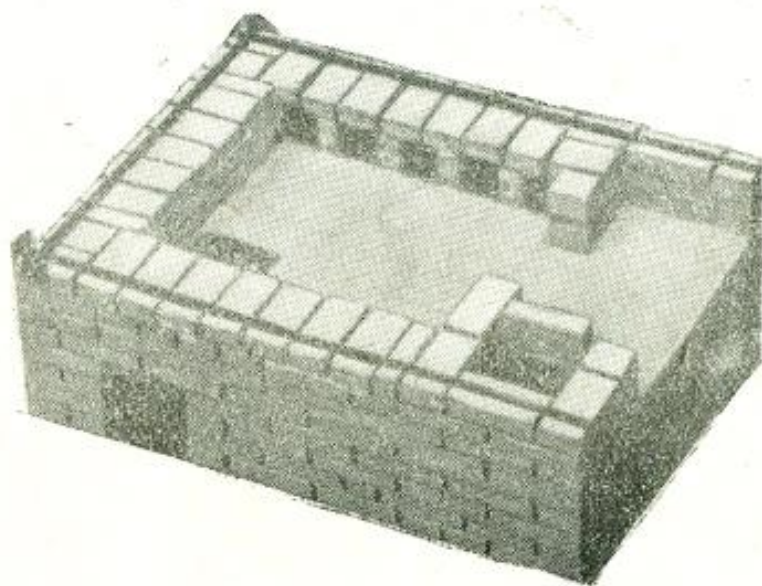
Рис. 99. Кладка 15-го ряда.
