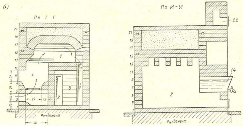
Рис. 14, б. Разрезы печи по Г-Г, И-И (см. рис. 12, а и б).
