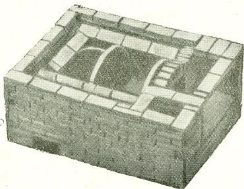
Рис. 33. Кладка 19-го ряда.
