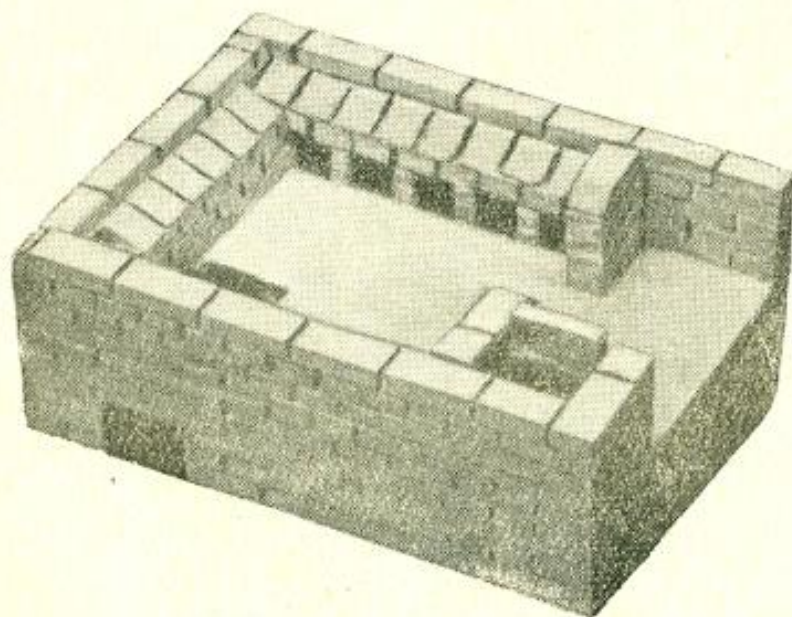
Рис. 31. Кладка 17-го ряда.
