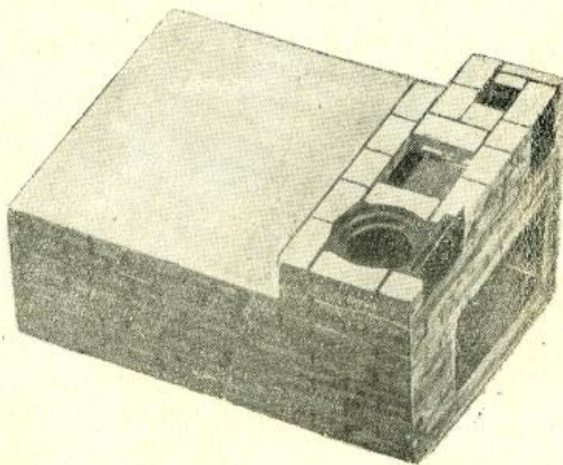
Рис. 39. Кладка 25-го ряда.
