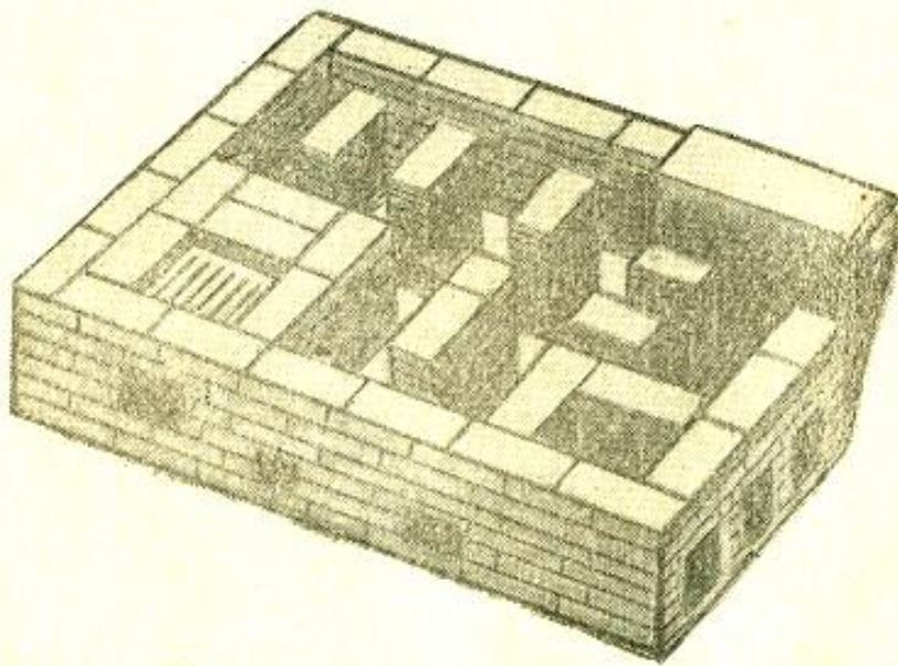
Рис. 20. Кладка 6-го ряда.
