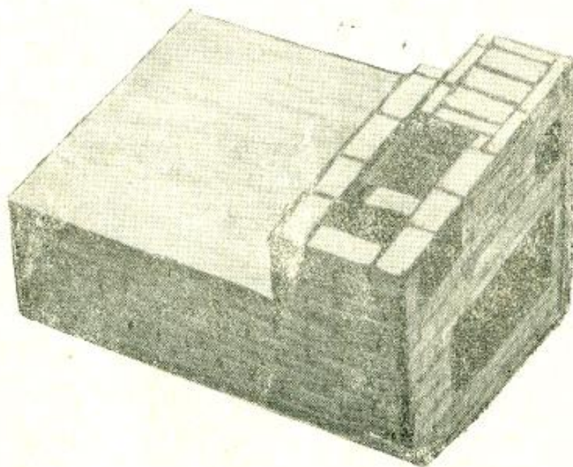
Рис. 41. Кладка 27-го ряда.
