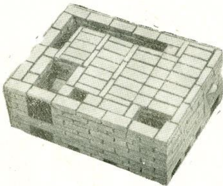
Рис. 25. Кладка 11-го ряда.
