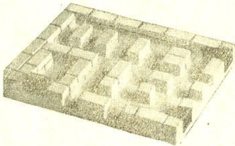
Рис. 17. Кладка 3-го ряда.
