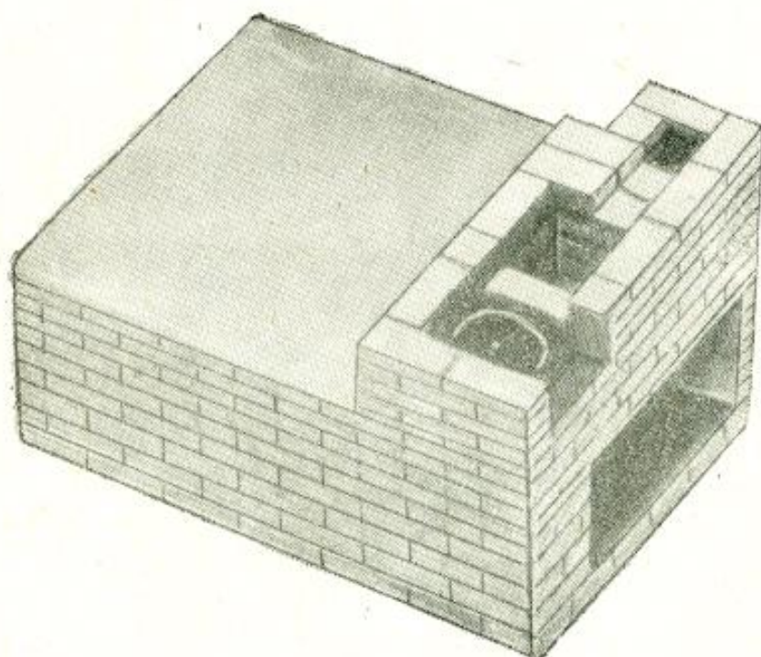
Рис. 40. Кладка 26-го ряда.
