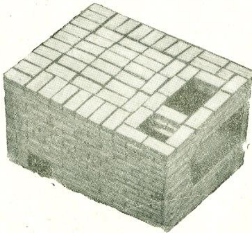
Рис. 36. Кладка 22-го ряда.
