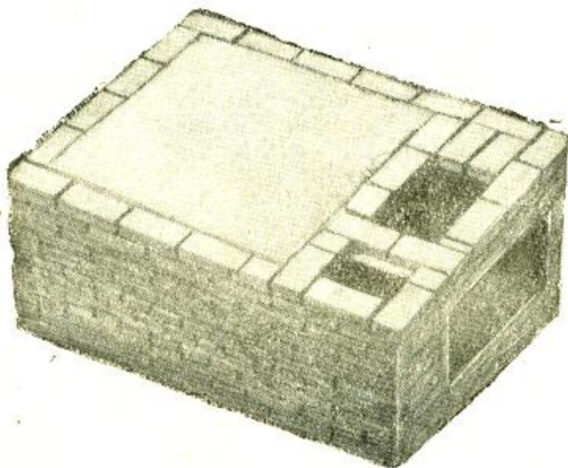
Рис. 35. Кладка 21-го ряда.
