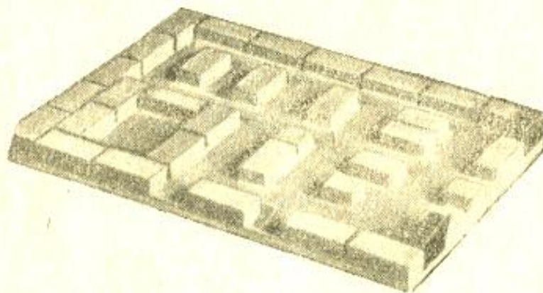
Рис. 16. Кладка 2-го ряда.
