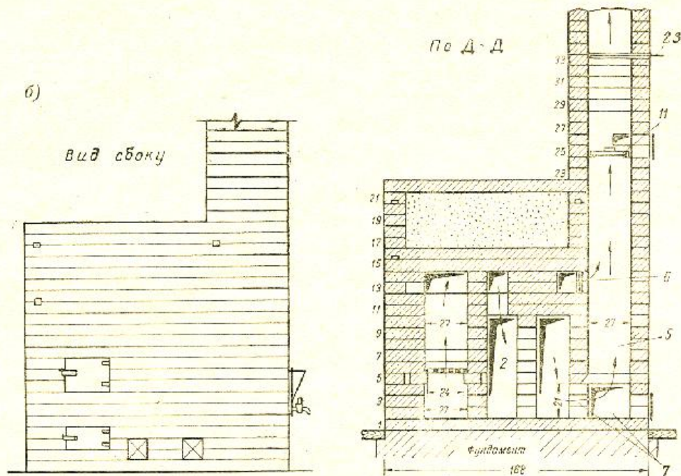
Рис. 13, б. Вид печи «Теплушка-2» сбоку и разрез по Д — Д (см. рис. 12, а и б).
