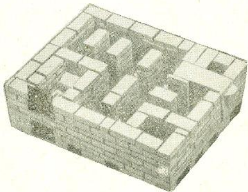
Рис. 23. Кладка 9-го ряда.
