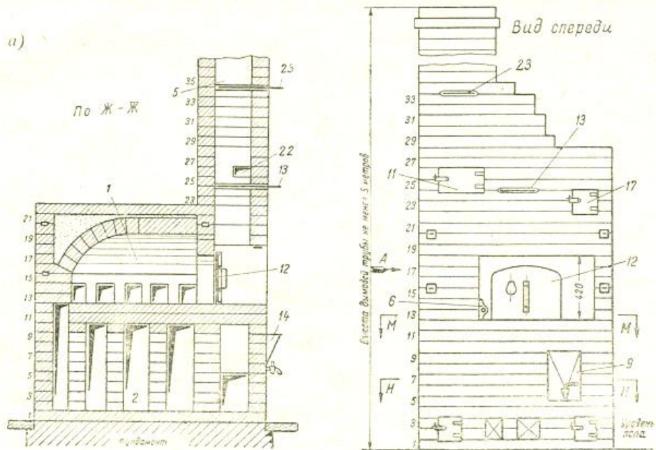
Рис. 13, а. Вид печи «Теплушка-2» спереди и разрез по Ж — Ж (см. рис. 12, а и б).
