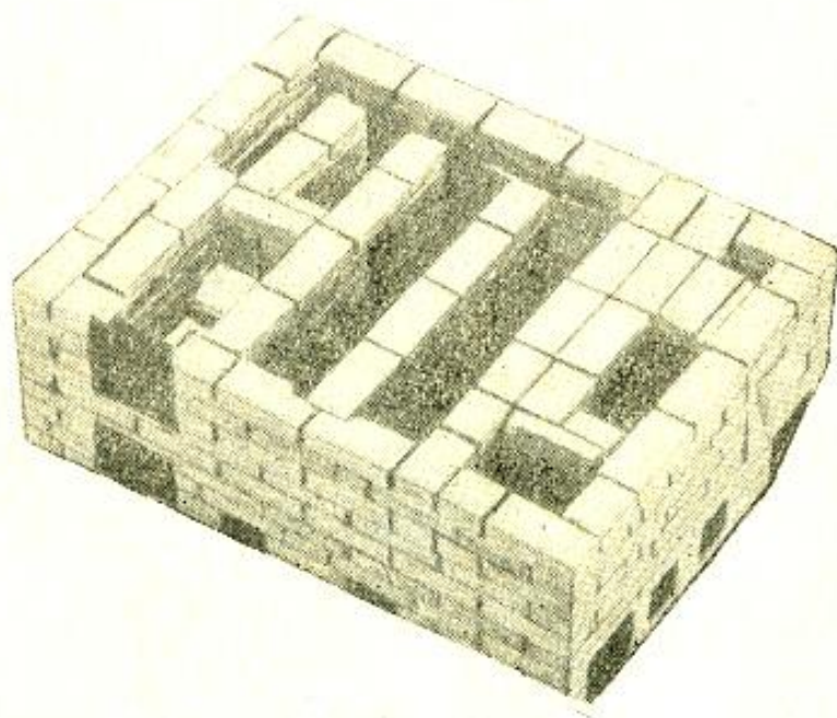
Рис. 24. Кладка 10-го ряда.
