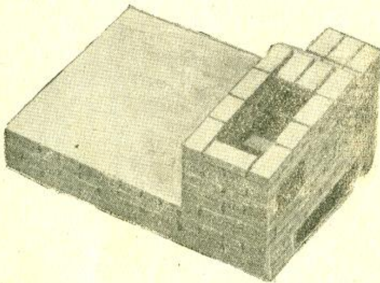
Рис. 43. Кладка 29-го ряда.
