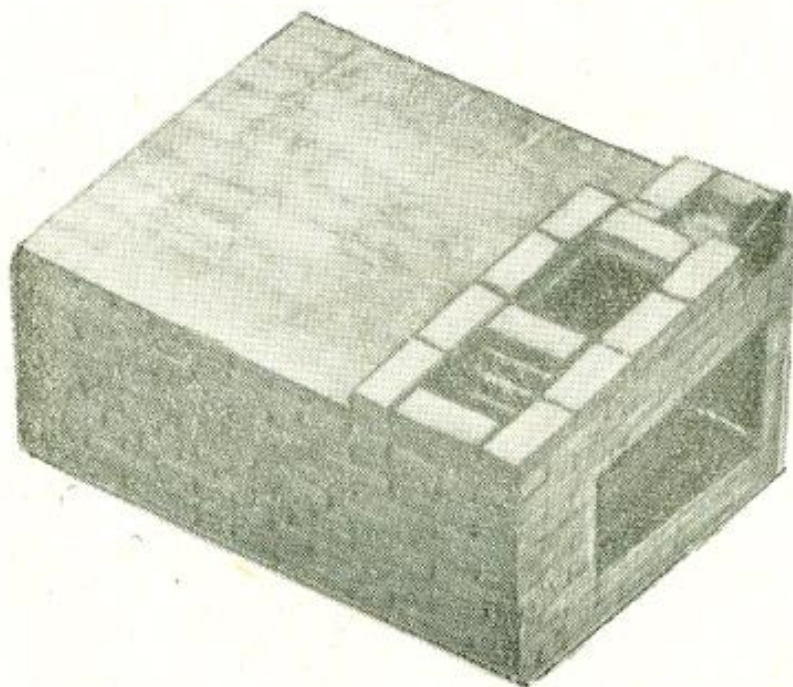
Рис. 37. Кладка 23-го ряда.
