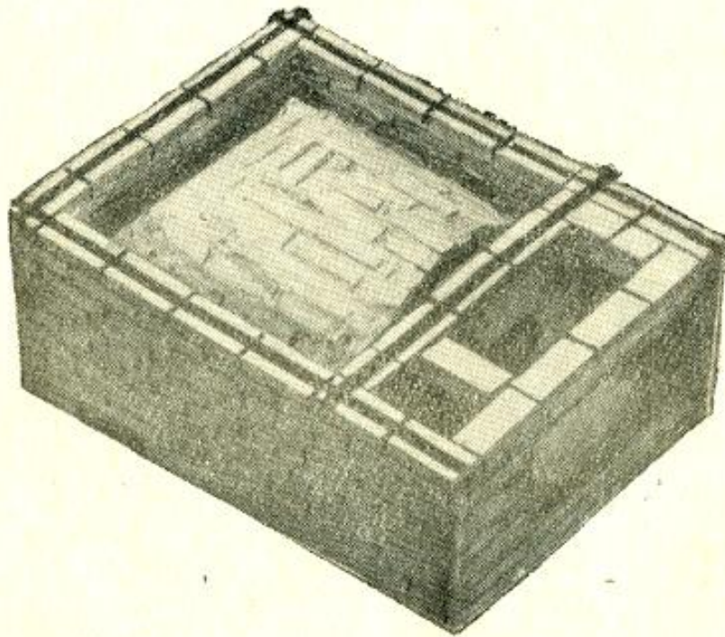
Рис. 34. Кладка 20-го ряда.
