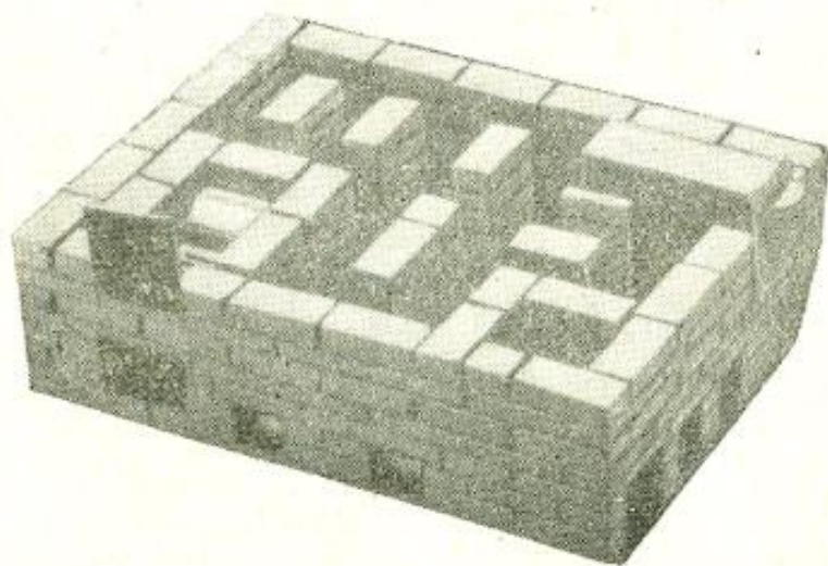
Рис. 22. Кладка 8-го ряда.
