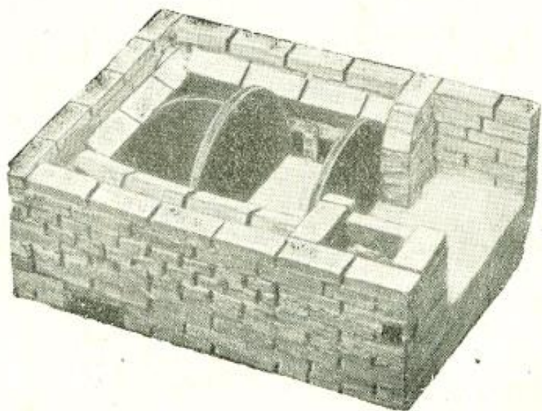
Рис. 32. Кладка 18-го ряда.
