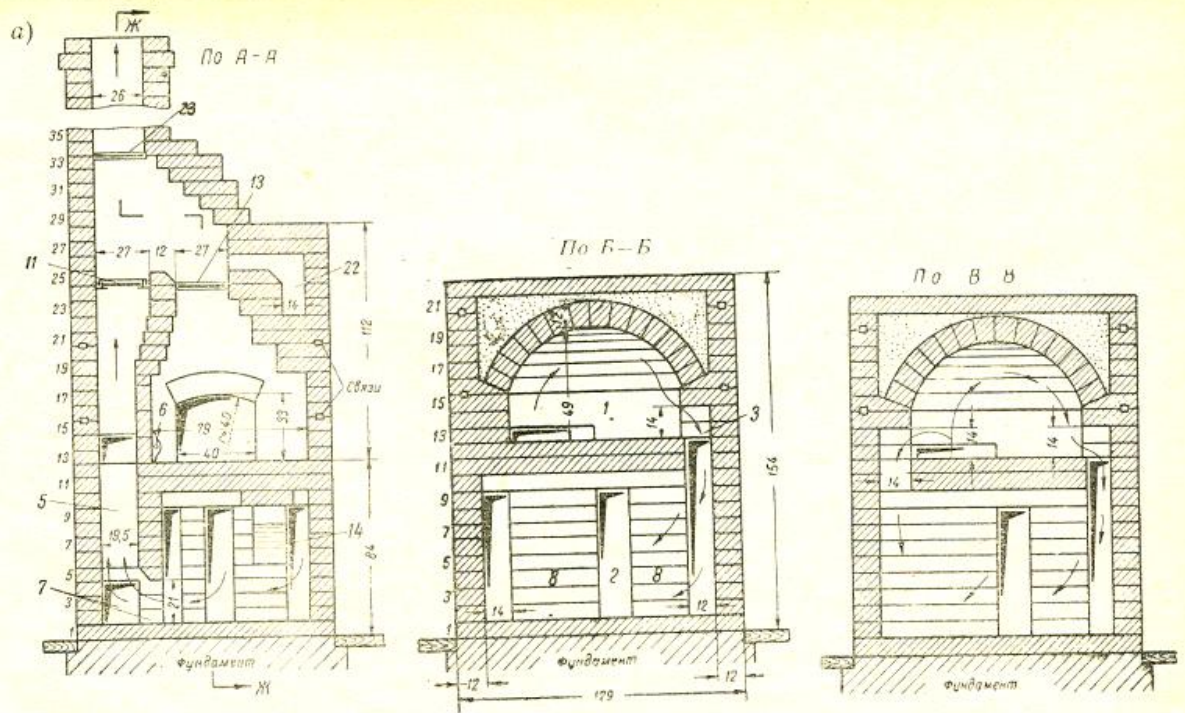
Рис. 14, а. Разрезы печи по А-А, Б-Б, В-В (см. рис. 12, а и б).
